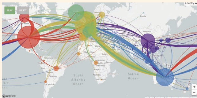
新型コロナウイルスの世界への伝搬状況 (7月2日現在:Nextstrain teamのホームページより)
